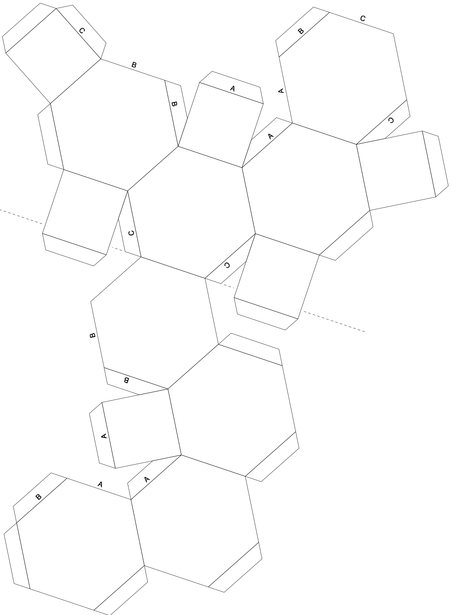
Stütz-Oktaeder (4,6,6) ( max. Kante = 3.0 cm )
