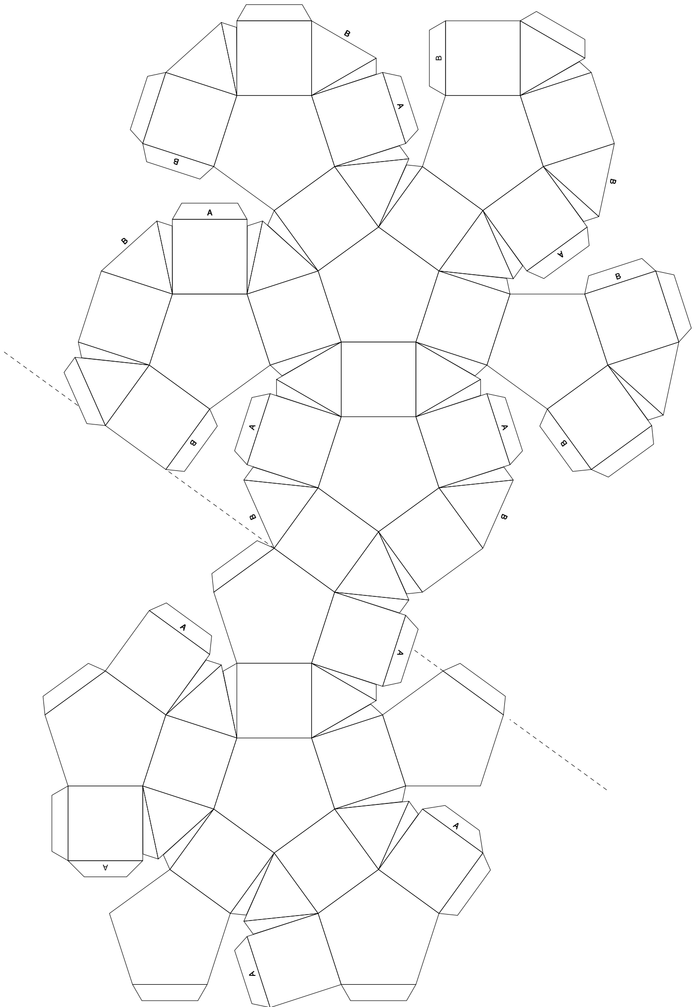
Klein-Rhombikosidodekaeder (3,4,5,4) ( max. Kante = 2.0 cm )
