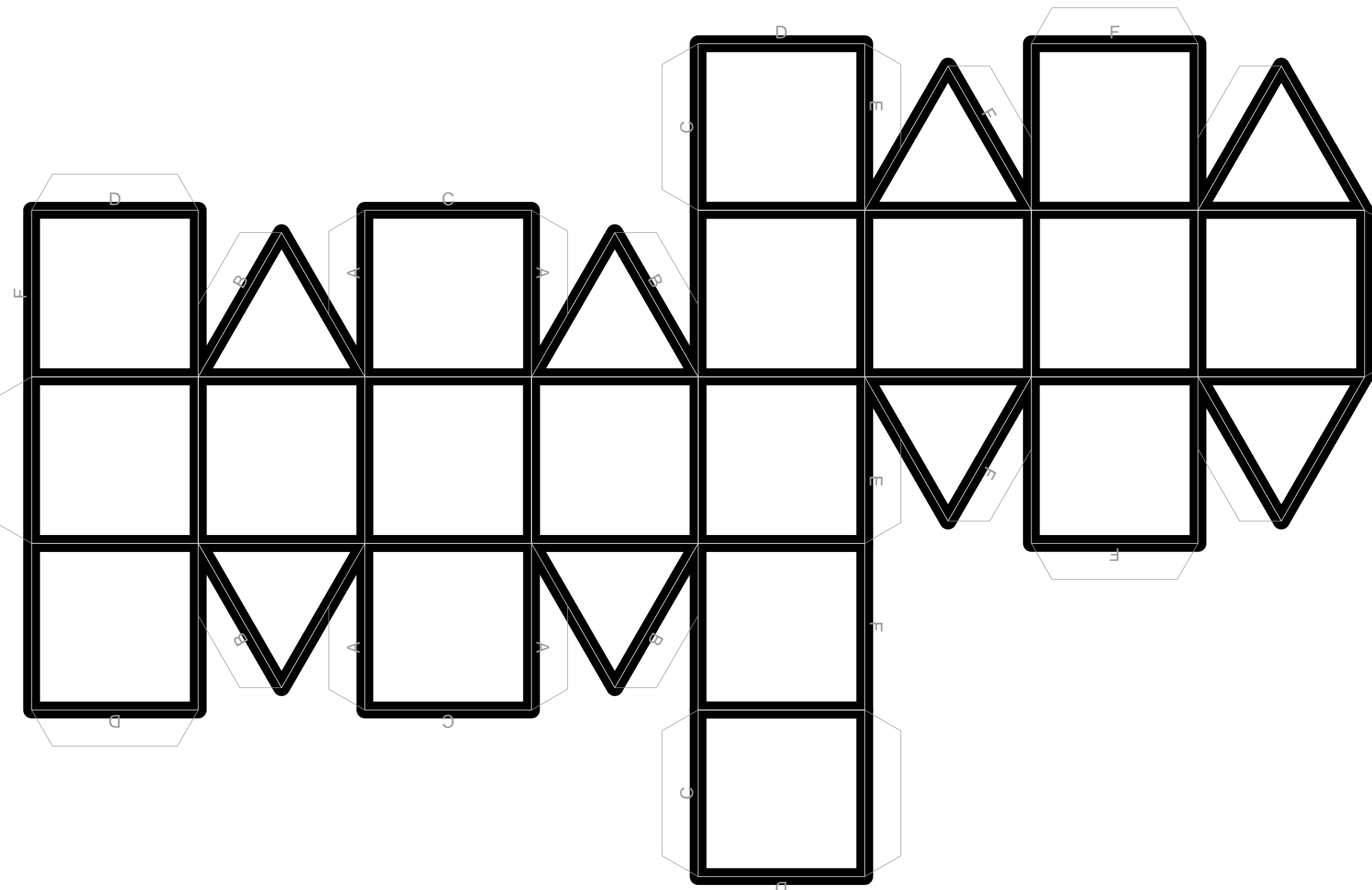
Pseudo-Rhombikuboktaeder (3,4,4,4)*
